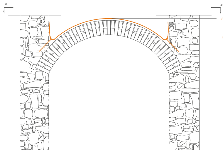
SEZIONE, SISTEMA DI RINFORZO ALL'ESTRADOSSO
