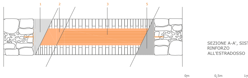
SEZIONE, SISTEMA DI RINFORZO ALL'ESTRADOSSO
